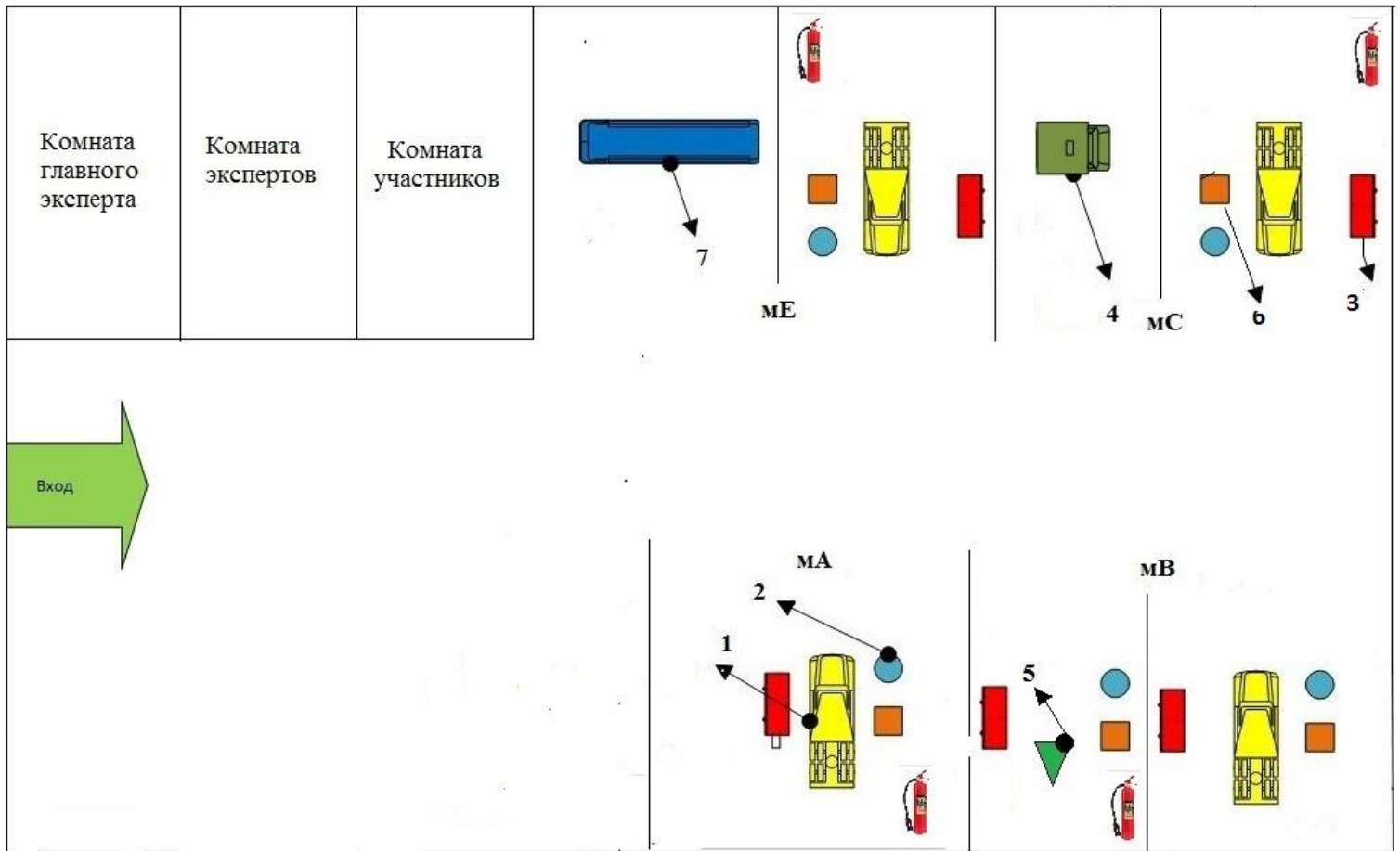
Схема расположения рабочих мест по модулям для проведения практических работ
